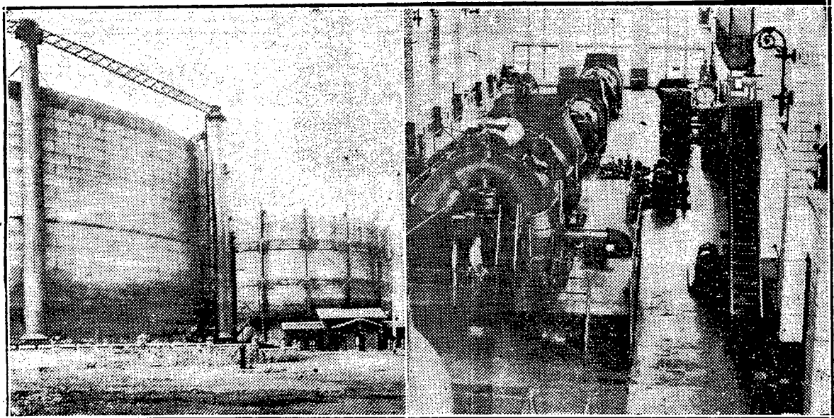
A la izquierda: la antigua fábrica de gas, que tan popular es a los habaneros; a la derecha: aspecto general de la Sala de Turbinas Generadoras (antigua) de la Planta de Tallapiedra, dotada de 12,500 kilowatts.
