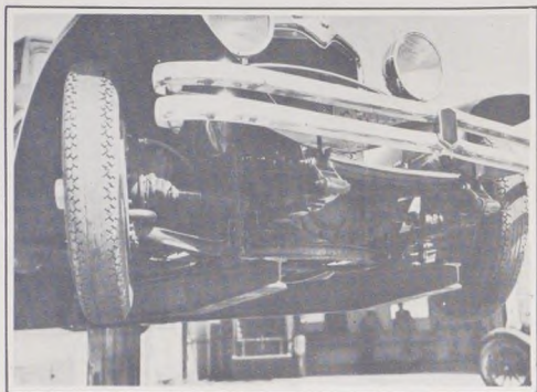
Frente del carro "Misterio" mostrando el diferencial en la parte delantera haciendo motrices las ruedas directrices.
