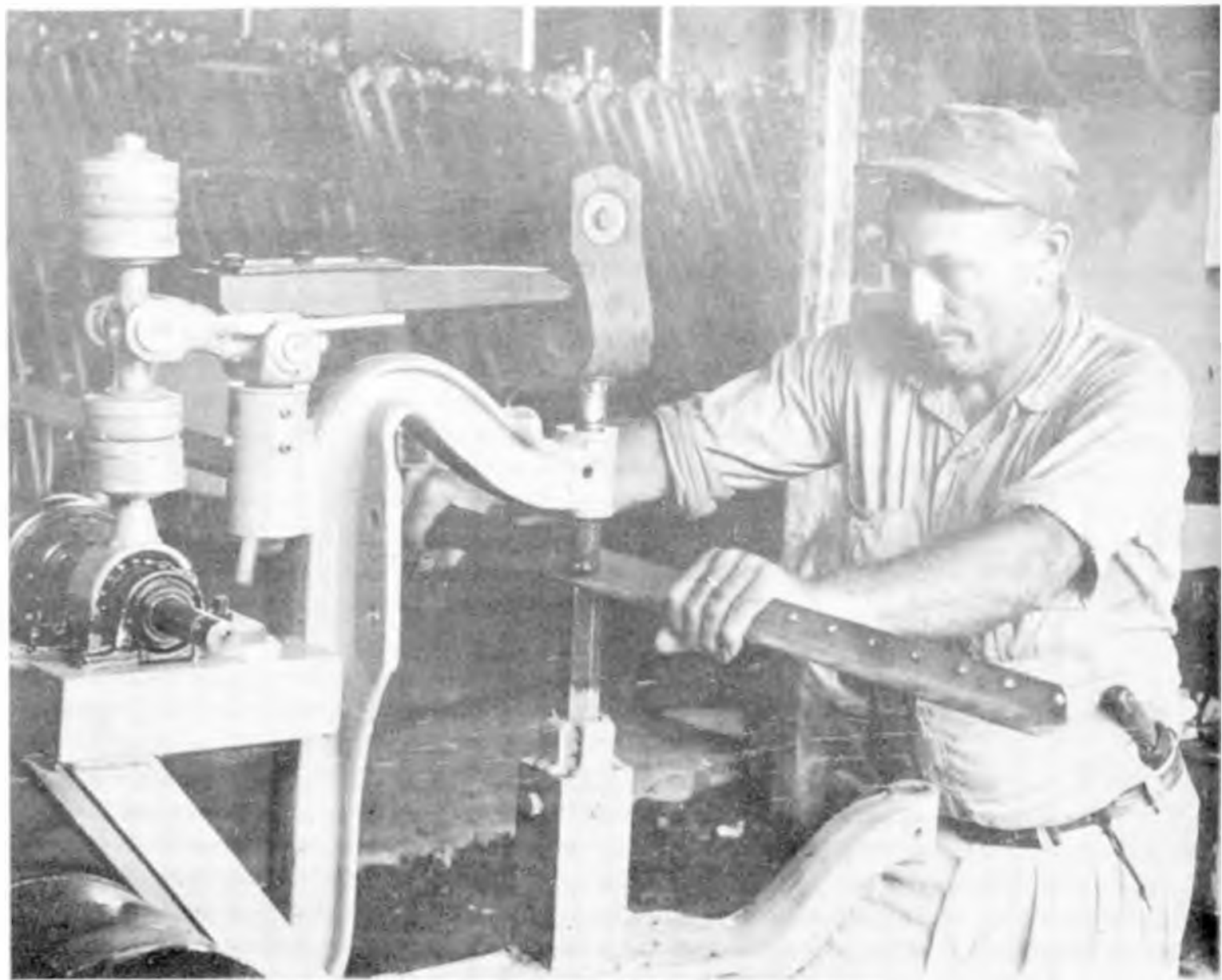
EL OPERARIO CELESTINO DELGADO COMPRUEBA LA EFICACIA DE ESTE OTRO REMACHADOR QUE TAMBIEN FUE CONSTRUIDO POR EL INGENIERO INDUSTRIAL CRIOLLO
